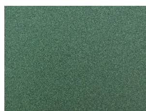
565 Σμαραγδί / Emerald
