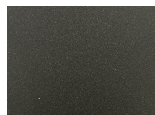
570 Άνθρακας / Carbon
