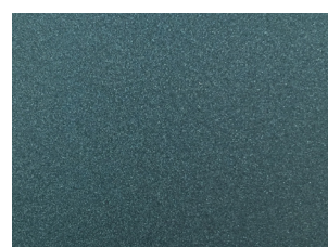
569 Αζουρίτης / Azurite
