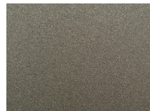
554 Οπάλιο / Opal
