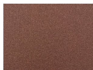
564 Ερυθρίτης / Erythrite
