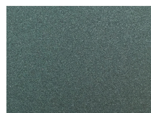
566 Ζαφείρι / Sapphire
