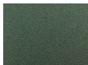
568 Αδαμίτης / Adamite
