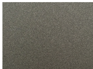
552 Μαγνητίτης / Magnetite
