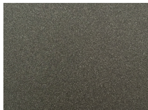
551 Γαλνίτης / Galena
