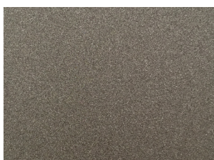
555 Λιθάργυρος / Litharge
