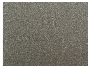
553 Δολομίτης / Dolomite
