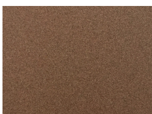
563 Χαλκός / Copper
